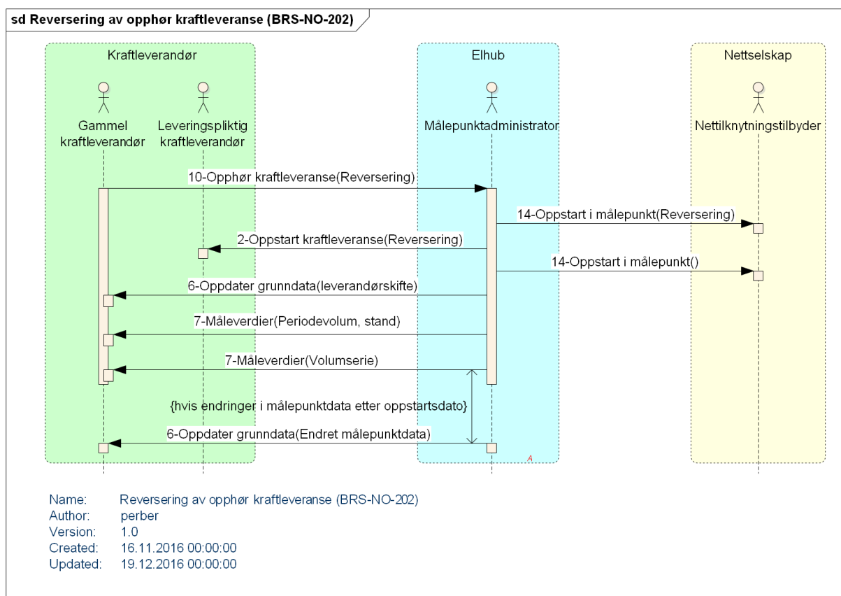
Figure 45 Sekvensdiagram Reversering av opphør kraftleveranse (BRS-NO-202)
