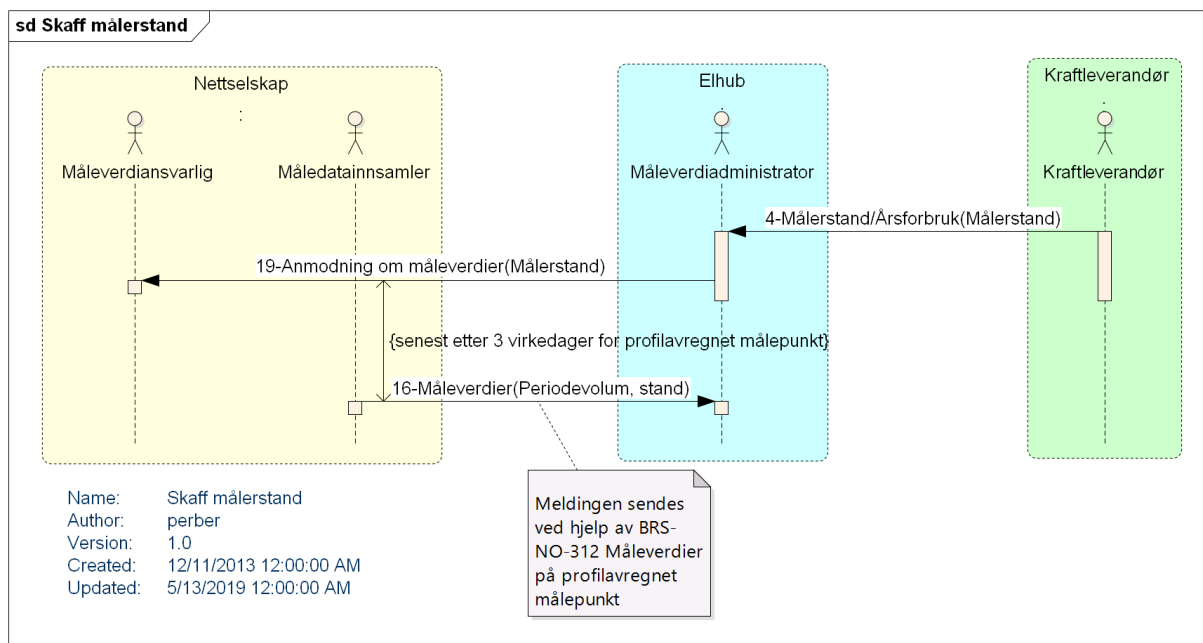
Figure 63 Sekvensdiagram for Målerstand fra kraftleverandør
