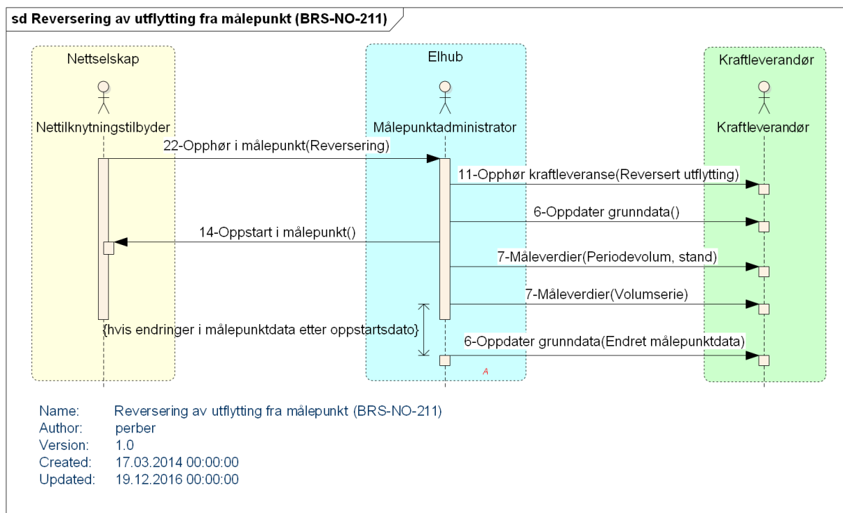
Figure 47 Sekvensdiagram Reversering av utflytting fra målepunkt
