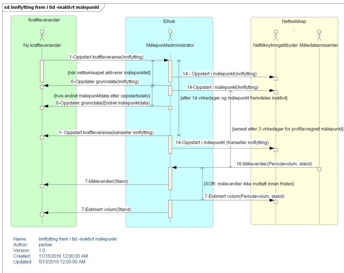
Figure 8 Sekvensdiagram for innflytting frem i tid -inaktivt målepunkt
