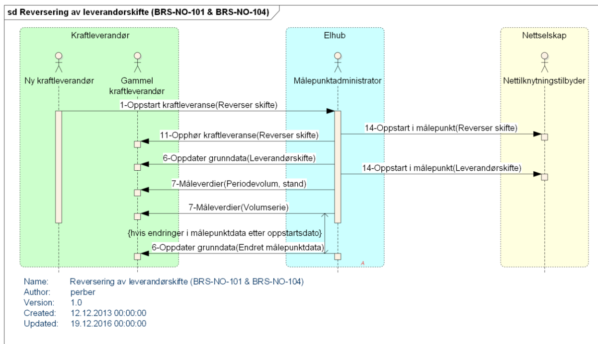
Figure 16 Sekvensdiagram Reversering av leverandørskifte (BRS-NO-101 &amp; BRS-NO-104)
