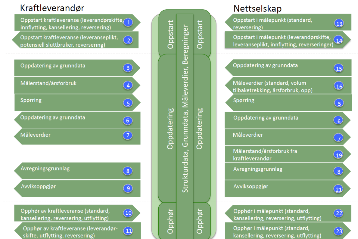
Figure 1 Meldinger/prosesskomponenter I
